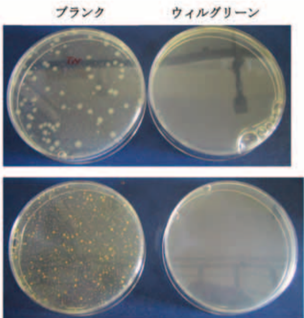
大腸菌
